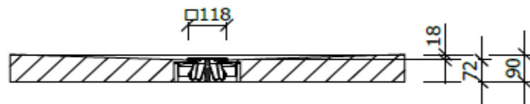
Schnitt A-A (1 : 15)
