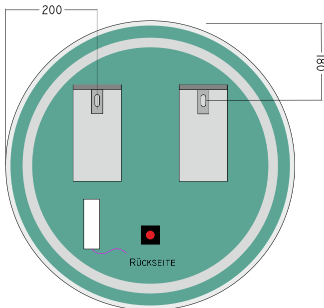
RÜCKANSICHT
