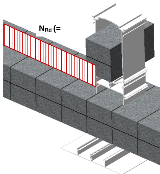
Abb. 9: Darstellung der Lasteinwirkung auf MSP-FR-EW-C
