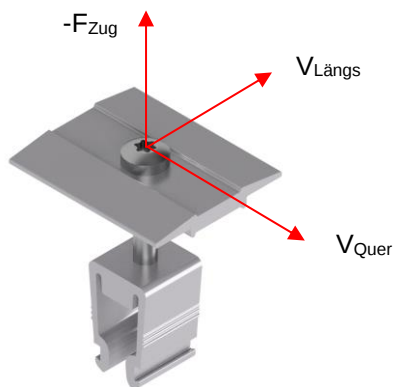
Abb. 6: Vektoren des Widerstands der MSP-PR-MCG Mittelklemme
