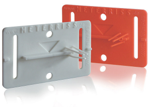
RS20 Meterriss-Plakette, zur dauerhaften Sicherung des Meterrisses bis nach den Putzarbeiten
