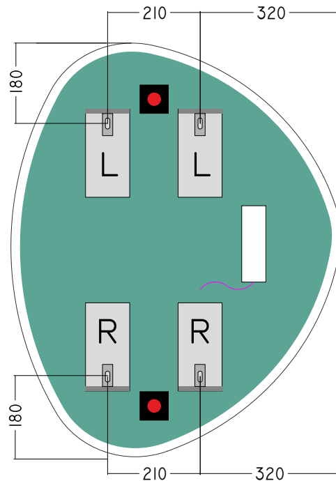
RÜCKANSICHT
