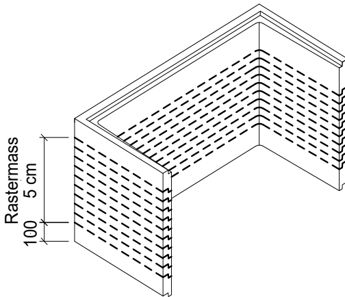
Bild 7: Zwischenhöhen
